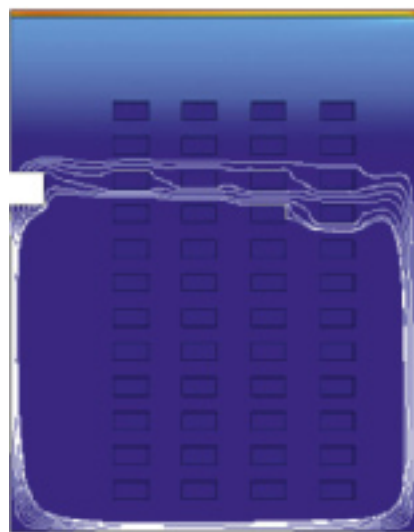
Figuur 4: Temperatuurprofiel in een vrieshuis. Bovenin is de lucht iets warmer. Uiteraard is deze berekening slechts een schets, en men kan met extra ventilatoren de lucht mengen en een homogenere temperatuur realiseren.
