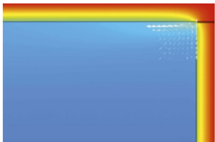
Figuur 5: Instroom van leklucht. De geïsoleerde wanden laten een warmtestroom door van ongeveer 6W/m 2 .
